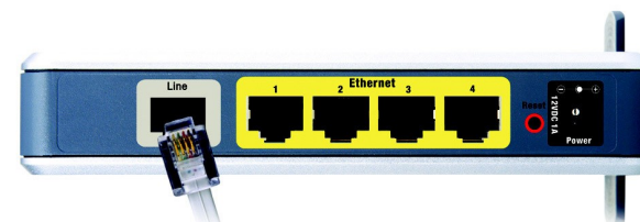
Rysunek 4-4: Podłącz linię ADSL
